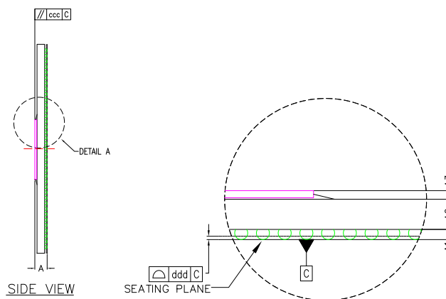
图 10.2 LS3A6000M 封装尺寸
